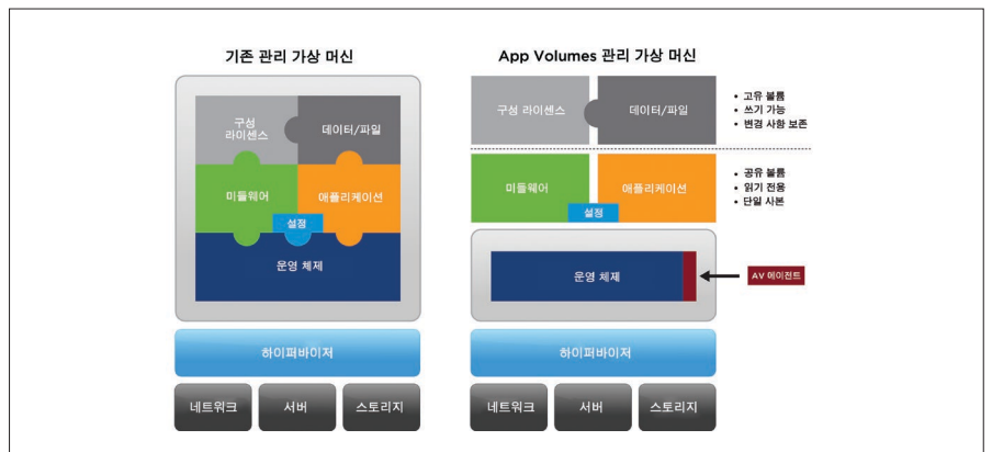
그림 4. App Volumes 관리 가상 머신이 OS보다 위에 가상화: 애플리케이션, 데이터 파일, 설정, 미들웨어 및 구성 라이선스가 별도의 계층 역할을 수행합니다.
